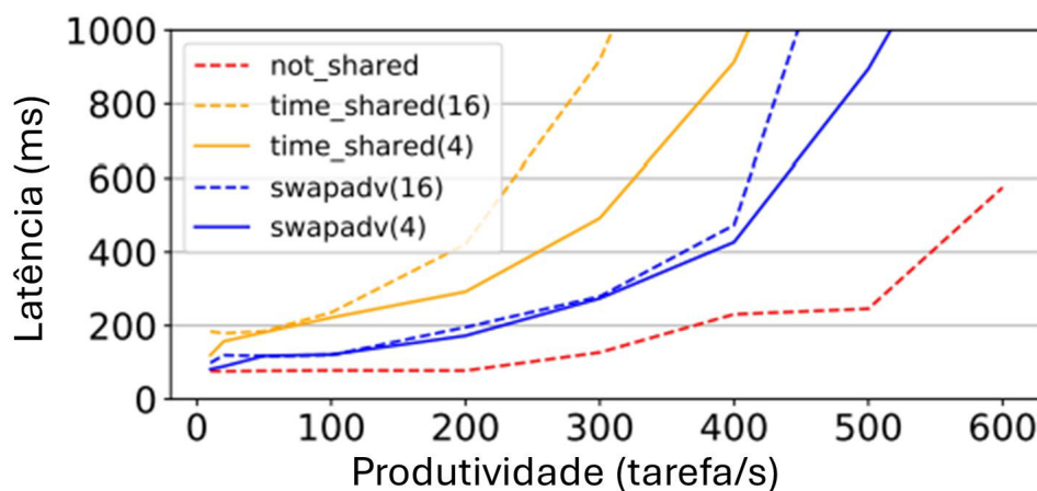
Figura 2. Latência de percentil 99 versus taxa de transferência para veiculação vários modelos ResNet-152. (Baseado em [ref]).
