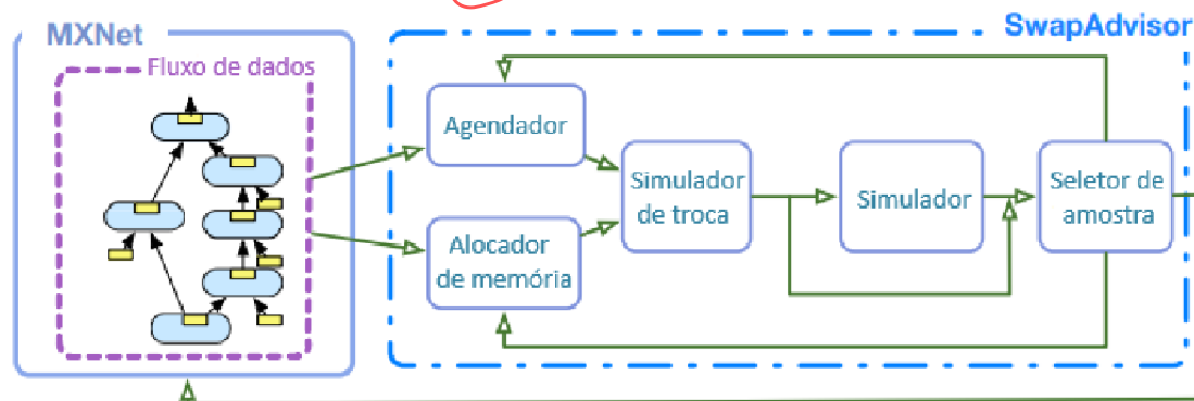
Figura 1. Visão geral do sistema do SwapAdvisor. (Baseado em [ref]).
